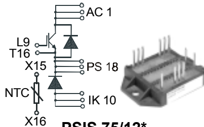
PSIS 75/12*
